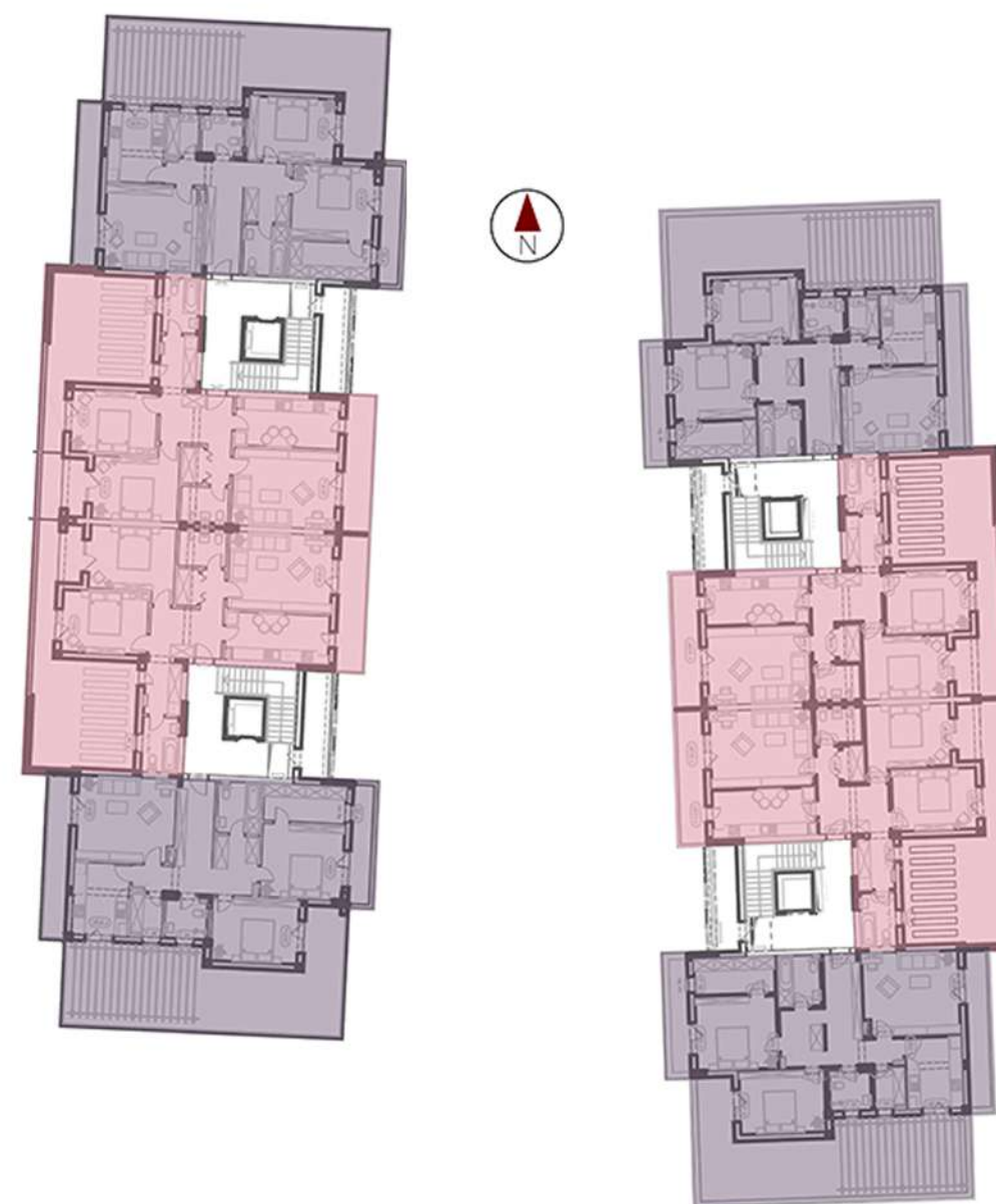
PLAN ETAJ 5
